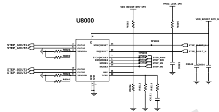
MOTOR
